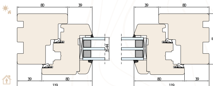
NATURO 80 SYSTEEM HORIZONTAAL DOORSNEDE B-B
