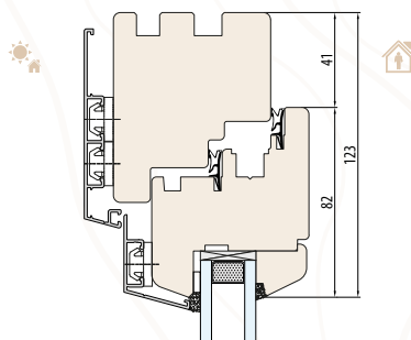
VERTICAAL DOORSNEDE A-A
